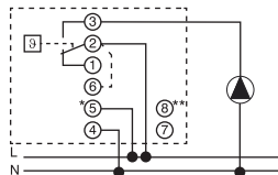
Commande d'un circulateur ou d'une vanne électrothermique
